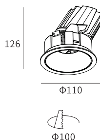
LLF320-12W Body Size : Ø110*126 Cut-Size : Ø100
