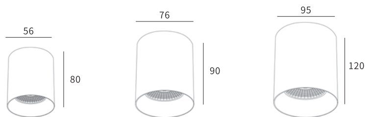
LLS124-7W Body Size :∅56*80
