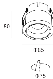
LLF310-15W Body Size : \varnothing 80*85 Cut-Size : \varnothing 75
