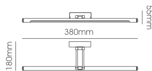
LLT012-5W Body Size: 380*180*55mm
