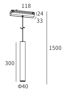
LMT 302 Body Size :Ø40*300
