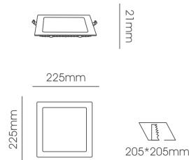
LLF055A-30W Body Size: 225*225*21mm Cut-Size: 205*205mm
