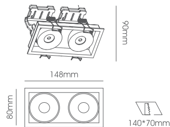
LLL065-18W Body Size: 148*80*90mm Cut-Size: 140*70mm
