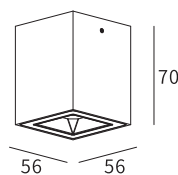
LLL 125-5W Body Size :56*56*70
