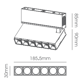
LLL019-6*2W Body Size: 185.5*30*175mm
