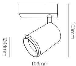
LLF224-6W Body Size: Ø44*103*103mm
