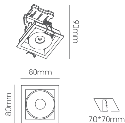
LLL064-9W Body Size: 80*80*90mm Cut-Size: 70*70mm
