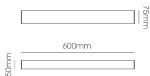
LLT036-25W Body Size: 600*50*75mm
