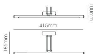
LLT014-5W Body Size: 415*185*100mm
