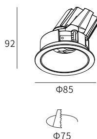
LLF319-9W Body Size : Ø85*92 Cut-Size : Ø75
