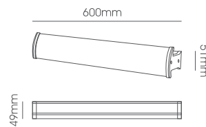
LLT027-15W Body Size: 600*49*51mm
