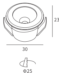
LLF093-1W Body Size : 30*H23mm Cut-Size : Ø25
