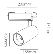
LLF159E/F-20/30W Body Size: Ø80*155*175*200mm
