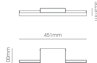
LLT020-8W Body Size: 451*100*50,5mm
