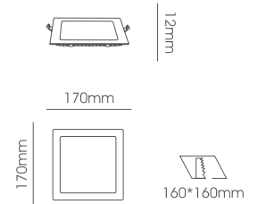
LLF014-12W Body Size: 170*170*12mm Cut-Size: 160*160mm
