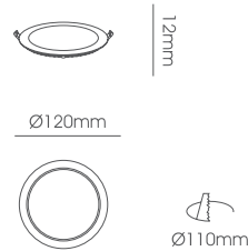
LLF008-9W Body Size: Ø120*12mm Cut-Size: Ø110mm
