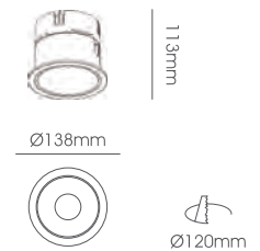
LLL100A-18W Body Size: Ø138*113mm Cut-Size: Ø120mm
