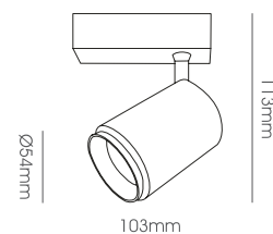
LLF225-12W Body Size: Ø54*103*113mm
