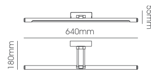
LLT013-12W Body Size: 640*180*55mm
