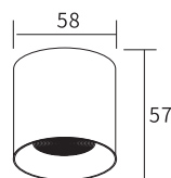
LLS 120(COB)-7W Body Size :Ø58*57
