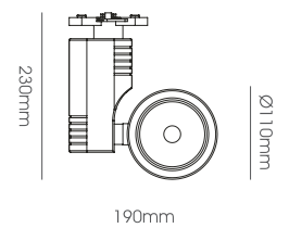
LLF151-30W Body Size: Ø110*190*230mm
