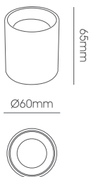
LLL011-7W Body Size: Ø60*65mm
